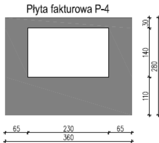
Rysunek 7 Płyta fakturowa P-4
