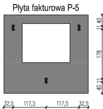
Rysunek 10 Schemat kotwienia płyty P-5
