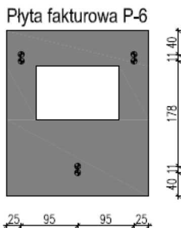
Rysunek 12 Schemat kotwienia płyty P-6
