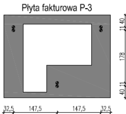
Rysunek 6 Schemat kotwienia płyty P-3
